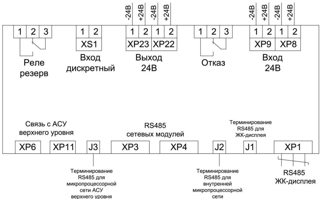
Рис. 2.Схема подключения блока сервера МСА.
