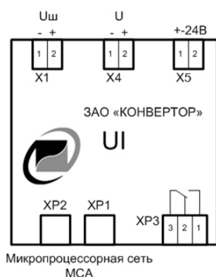
Рис. 5. Схема подключения модуля UI (где U— измеряемое напряжение; U ш - измеряемое напряжение шунта).
