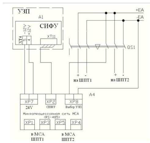
Рис. 28. Схема подключения модуля выбора ЩПТ (где А4 — модуль выбора УЗП; QS1 — рубильник АВВ OT125F3C)
